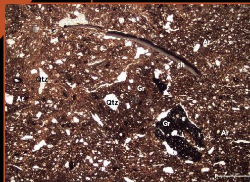
Vékonycsiszolat Vattina kerámiából, Omoljica lelőhelyről. Agyag (Ar), tört kerámia (grog) (Gr), kvarc (Qtz) és bioklaszt (Sh)
