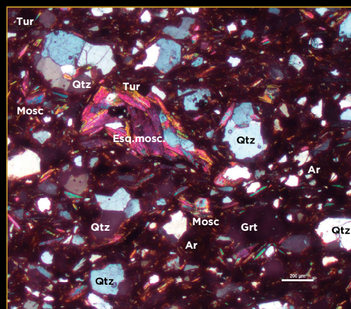
Kerámia vékonycsiszolat polarizációs mikroszkóp alatt készült képe. Agyag (Ar) kvarc (Qtz); moszkovit pala (Esq. mosc.); gránit (Grt); moszkovit csillámpala (Mosc); turmalin (Tur). Nagyítás: 0,2 mm
